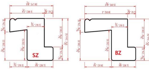
Small Z Frame (SZ)
