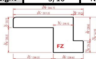
Flat Z (FZ)
