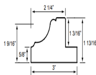
3" Deco Frame (DFO)
