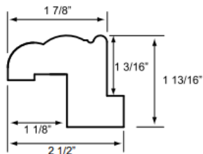
Matagorda Z-Frame (MAZ)
