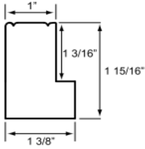
L-Frame (LFI, LFO)
