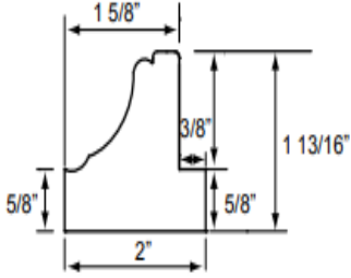
Deco Frame (D2O)
